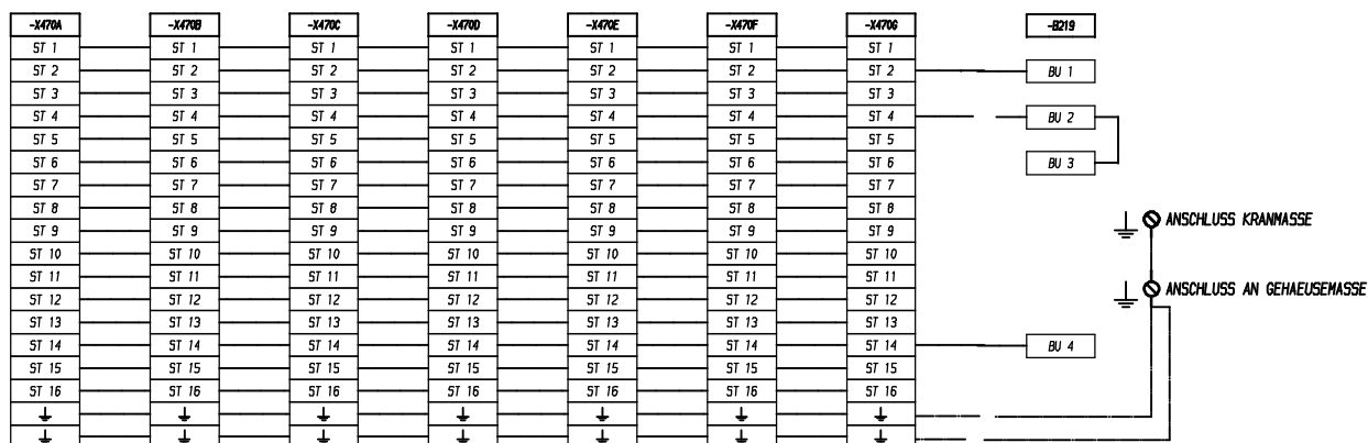
ANSCHLUSSBILD
